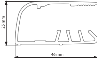
DESIGN PURE YP Dönüş Profili
