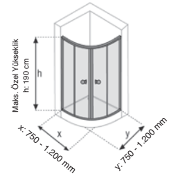
Standart Yükseklik h: 190 cm
