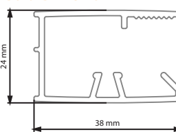
SOLVA SAK - DESIGN PURE SAK Duvar Dikme Profili
