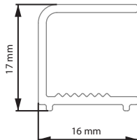
AURA KY SOLVA MİNİMAL Kuvet Üzeri Yp Dönüş Profili
