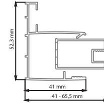
8mm Duvar Dikme Profili
