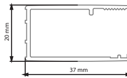
XTENSA Duvar Dikme
