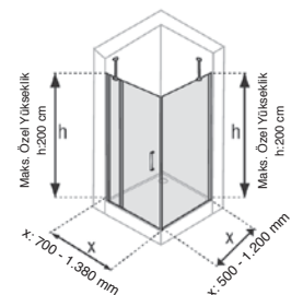
Standart Yükseklik h: 190 cm
