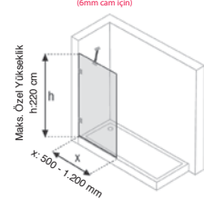
Standart Yükseklik h: 200 cm (6mm cam için)
