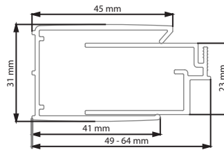
SOLVA AK Duvar Dikme ve Ayar Profili
