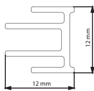
SOLVA MİNİMAL AK SAK Kapı Karşılığı Profili
