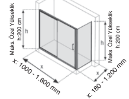
Standart Yükseklik h: 150 cm
