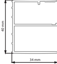
X1 - X0 - CLASSICS PS X1 EASY ENTRY Duvar Dikme Ayar Profili
