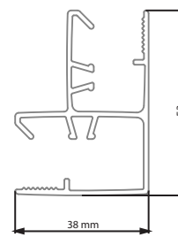
SOLVA MİNİMAL AK Duvar Dikme Profili
