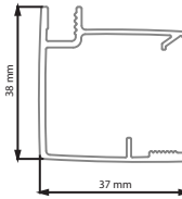
SOLVA SAK - DESIGN PURE SAK Duvar Dikme Profili
