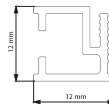
SOLVA MİNİMAL AK Duvar Dikme Profili
