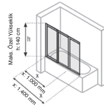
Standart Yükseklik h: 140 cm
