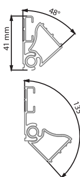
Mafsallı Profil Seti
