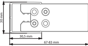
DESIGN PURE AK Duvar Dikme Ayar Profili
