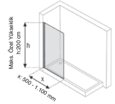
Standart Yükseklik h: 150 cm
