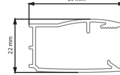
CLASSICS KY C YP T Duvar Dikme
