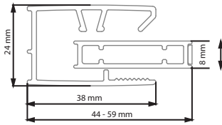
SOLVA AK SAK Kapı Karşılığı Profili
