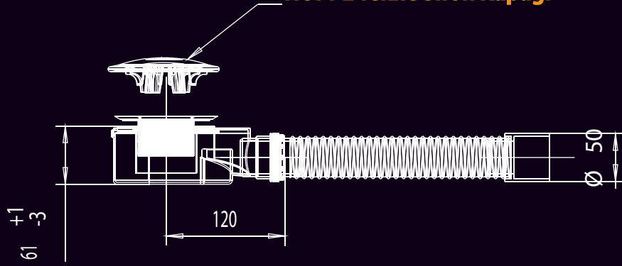
HÜPPE Tekne Sifon Kapağı
