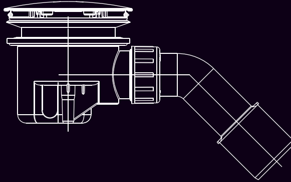
Viega Tekne Sifon Seti
