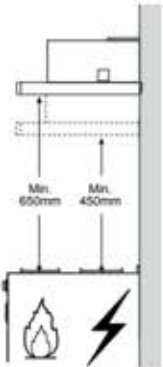
Sürgülü Aspiratör
