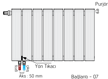
Bağlantı - 07 ( Sol giriş çıkışlı kompakt bağlantı. )
