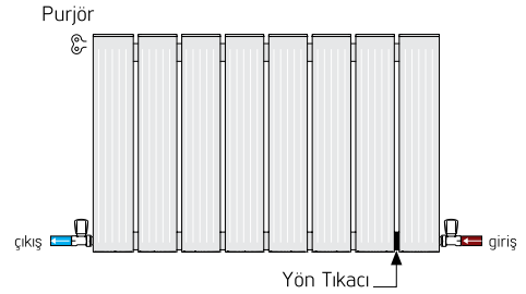
Bağlantı - 04 ( Alt sağ giriş alt sol çıkış alt karşıt bağlantı. )
