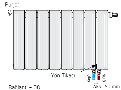
Bağlantı - 08 ( Sağ giriş çıkışlı kompakt bağlantı. )
