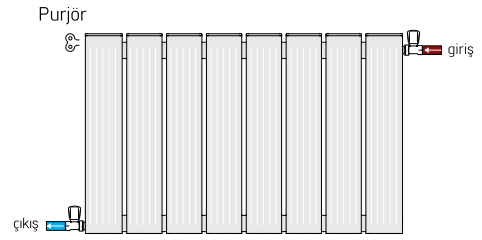
Bağlantı - 06 ( Üst sağ giriş alt sol çıkış çapraz bağlantı. )
