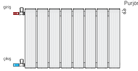
Bağlantı - 01 ( Üst sol giriş alt sol çıkış paralel bağlantı. )
