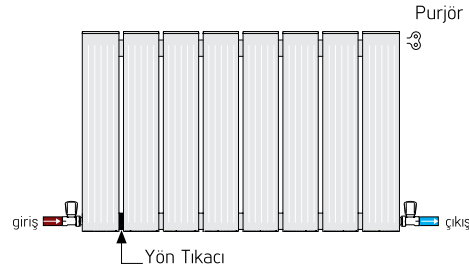
Bağlantı - 03 ( Alt sol giriş alt sağ çıkış alt karşıt bağlantı. )
