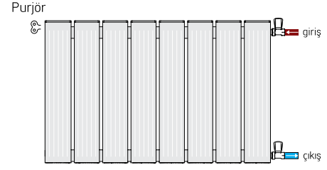
Bağlantı - 02 ( Üst sağ giriş alt sağ çıkış paralel bağlantı. )
