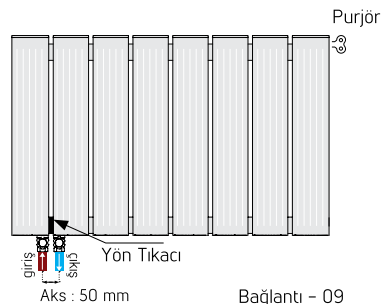
Bağlantı - 09 ( Sol giriş çıkışlı hb bağlantı. )
