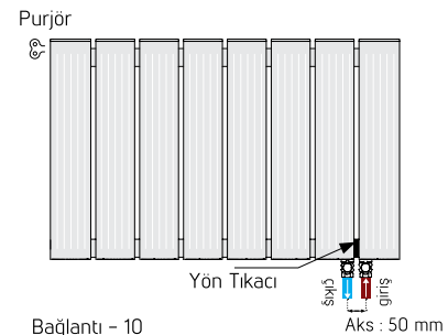
Bağlantı - 10 ( Sağ giriş çıkışlı hb bağlantı. )
