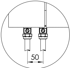
Mini Küresel Vanalı Bağlantı
