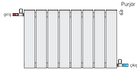
Bağlantı - 05 ( Üst sol giriş alt sağ çıkış çapraz bağlantı. )
