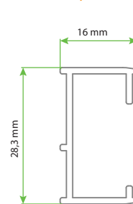
X1 PLATFORMU - DESIGN AK DESIGN SAK - DESIGN AKT AURA SAK 1,5 CM Uzatma Profili
