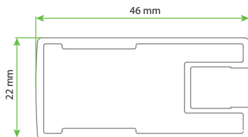
AURA KY SOLVA YP Dönüş Profili
