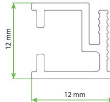
SOLVA MİNİMAL AK Duvar Dikme Profili
