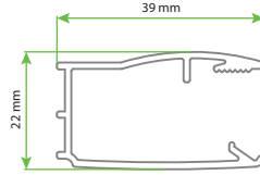
CLASSICS KY C Y P T Duvar Dikme
