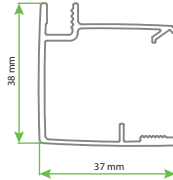
SOLVA SAK - DESIGN PURE SAK Duvar Dikme Profili
