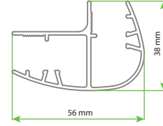
X1 - X0 - CLASSICS PS X1 EASY ENTRY Duvar Dikme Ayar Profili
