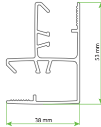
SOLVA MİNİMAL AK Duvar Dikme Profili
