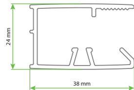
SOLVA SAK - DESIGN PURE SAK Duvar Dikme Profili
