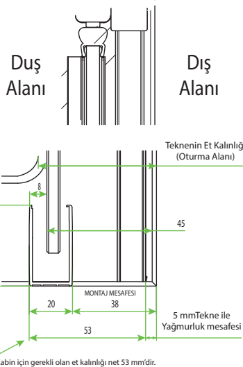
TEK KANALLI DUVAR DİKME PROFİLİ
