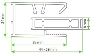
SOLVA AK SAK Kapı Karşılığı Profili
