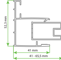
8mm Duvar Dikme Profili
