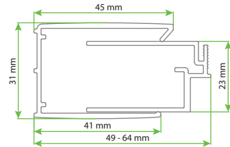
SOLVA AK Duvar Dikme ve Ayar Profili
