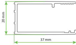
XTENSA Duvar Dikme
