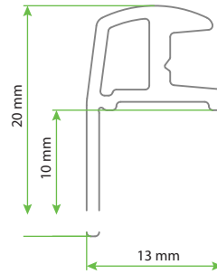
XTENSA AQUANIT TEKNE için ön cephe - köşe giriş alt ray profili
