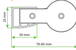
DESIGN AK - DESIGN AKT Duvar Dikme Ayar Profili
