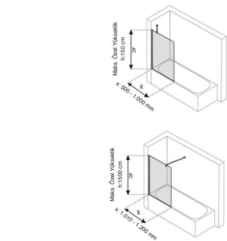
Opsiyonel: D tipi cam
