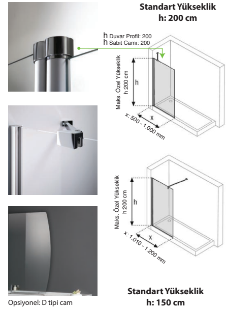
Opsiyonel: D tipi cam
