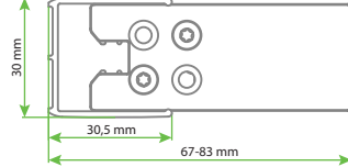
DESIGN PURE AK Duvar Dikme Ayar Profili
