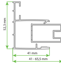
X1 - X0 - CLASSICS PS X1 EASY ENTRY Kulaklı Duvar Dikme Ayar Profili
