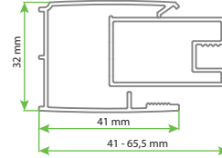
X1 - X0 - CLASSICS PS X1 EASY ENTRY Duvar Dikme Ayar Profili
