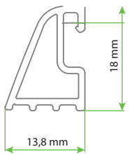
XTENSA AQUANIT Tekne için Yan Panel Alt Ray Profili
