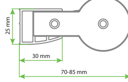
DESIGN AK - DESIGN AKT Duvar Dikme Ayar Profili
