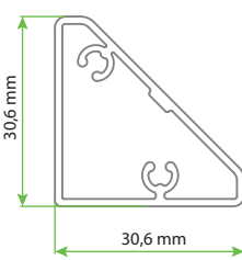
X1 - X0 - CLASSICS PS ST - PT Çerçeve Profili
