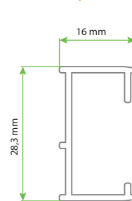
X1 PLATFORMU - DESIGN AK DESIGN SAK - DESIGN AKT AURA SAK 1,5 CM Uzatma Profili
