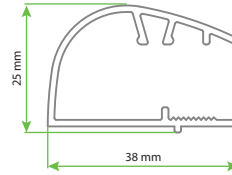
DESIGN AK YP Dönüş Profili
