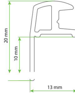
XTENSA AQUANIT TEKNE için ön cephe - köşe giriş alt ray profili
