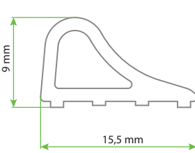
XTENSA AQUANIT Tekne için Yan Panel Alt Ray Profili
