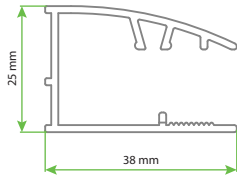
DESIGN - AURA SAK Duvar Dikme
