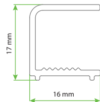
AURA KY SOLVA MINIMAL Kuvet Üzeri Yp Dönüş Profili XTENSA YP (K2S2 - K1S2 UY.)
