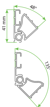
Mafsallı Profil Seti
