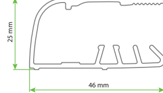
DESIGN PURE YP Dönüş Profili
