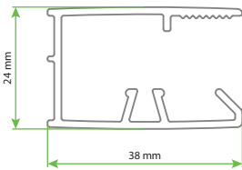
DESIGN PURE SAK Duvar Dikme Profili
