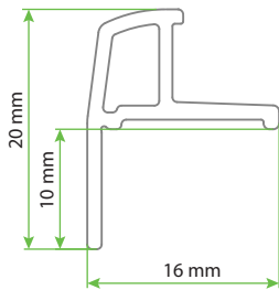
XTENSA AQUANIT Tekne için Yan Panel Alt Ray Profili
