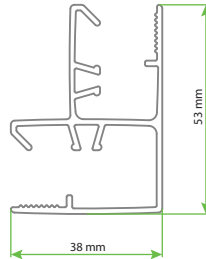
AURA KY SOLVA YP Dönüş Profili
