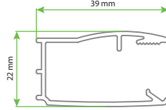
CLASSICS KY C YPT Duvar Dikme
